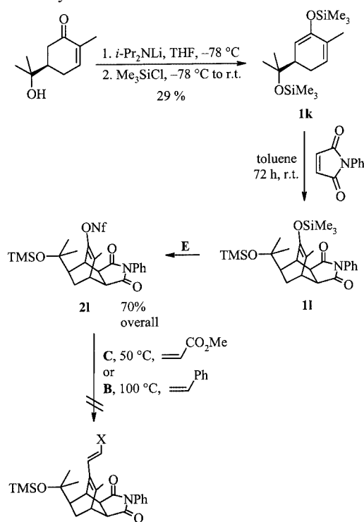
Scheme 12. B : Pd(OAc) 2 , KOAc, K 2 CO 3 , DMF, 24 h; C : Pd(OAc) 2 , LiCl, Et 3 N, DMF, 20 h; E : dibenzo-18-crown-6, KF, NfF, DMF/THF, room temp., 67 h
