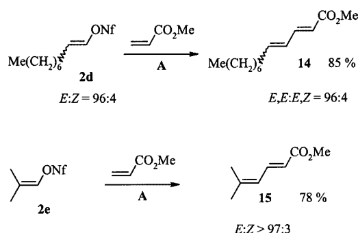
Scheme 4. A: Pd(OAc) 2 , n Bu 4 NCl, K 2 CO 3 , DMF, room temp., 6 h
